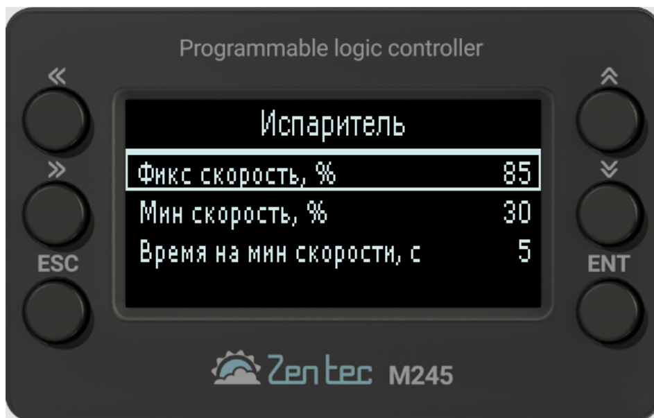
Рис. 8 Меню вентилятора в режиме сервиса
